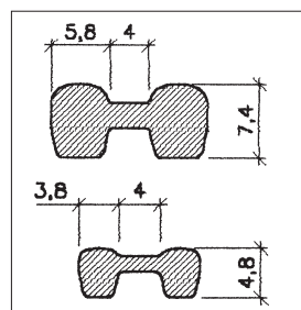
Trådtverrsnitt
