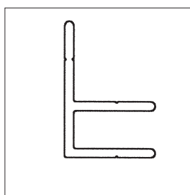
Profilnavn: Amplinet omramming Profilnr.: 321097 Produktnr.: 242053 0520 242053 0525 eloksert Katalogside: 46
