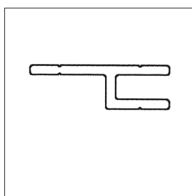
Profilnavn: Amplinet omram.prof Profilnr.: 321100 Produktnr.: 242053 0537 Katalogside: 47
