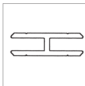
Profilnavn: Amplinet H-profil Profilnr.: 321102 Produktnr.: 242053 0560 Katalogside: 47
