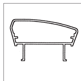
Profilnavn: Håndløberprofil Profilnr.: 4T-709 Produkt nr.: 241395 0345 Katalogside: 57
