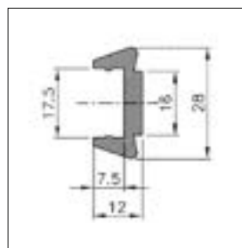
Profilnavn: Skruholderprofil Profilnr.: K16241 Vekt: 0,44kg/m Passer for skrue M10 For K19378 og 4T-832
