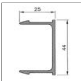
Profilnavn: Dekklisprofil Profilnr.: K16240 Vekt: 0,48 kg/m
