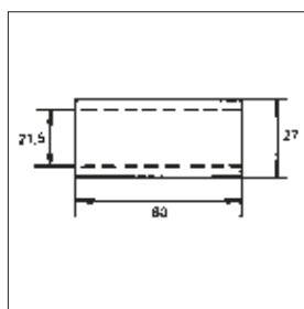
Lagerhylse, stål
