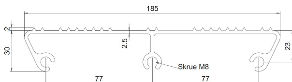
Trinnprofil 185 mm
