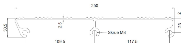
Trinnprofil 250 mm
