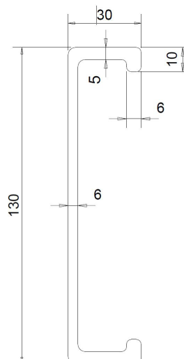
Vangeprofil 130 mm
