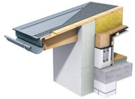
Fig. 2: Ikke ventilert takkonstruksjon med strukturmatte
